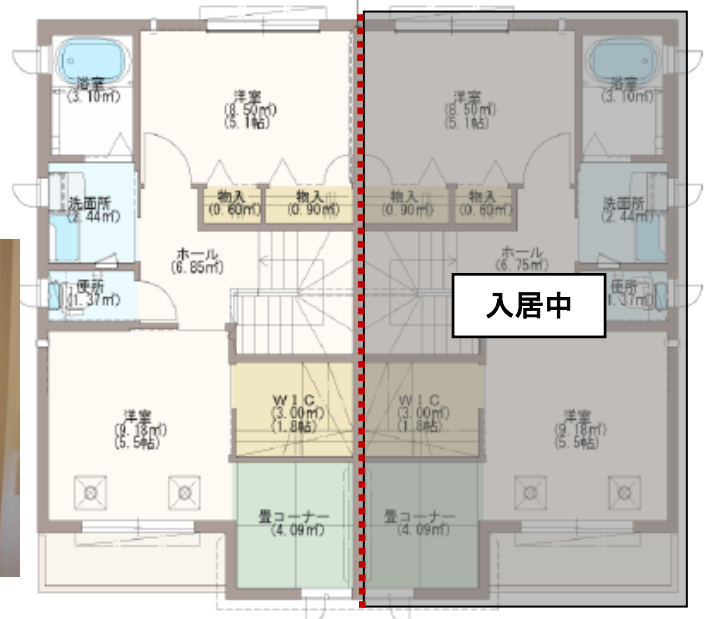
2号 2階平面図 1号
