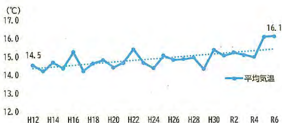
図 3.42 気温の推移
