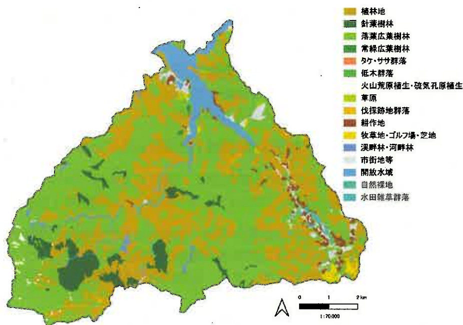
図 3.11 植生図
