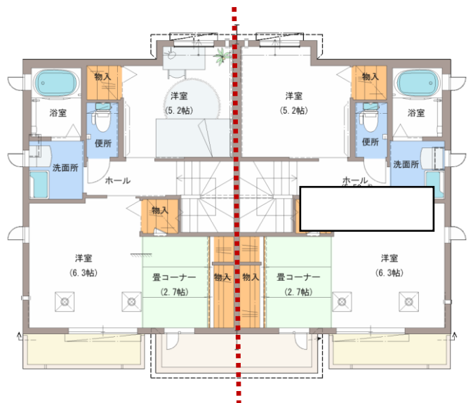
2号 2階平面図 1号
